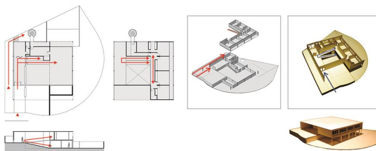
Figura 19: Análise da circulação e percurso num projeto não construído. Residência José David Vicente (1959). Arquitetos Vilanova Artigas e Carlos Cascardi.
