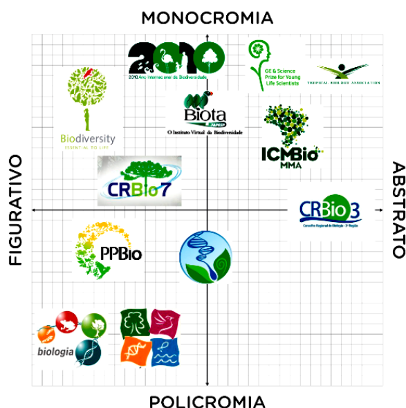
Figura 5: Diagrama Semântico.
